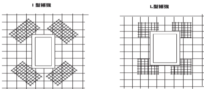
◇開口部補強メッシュ使用例
